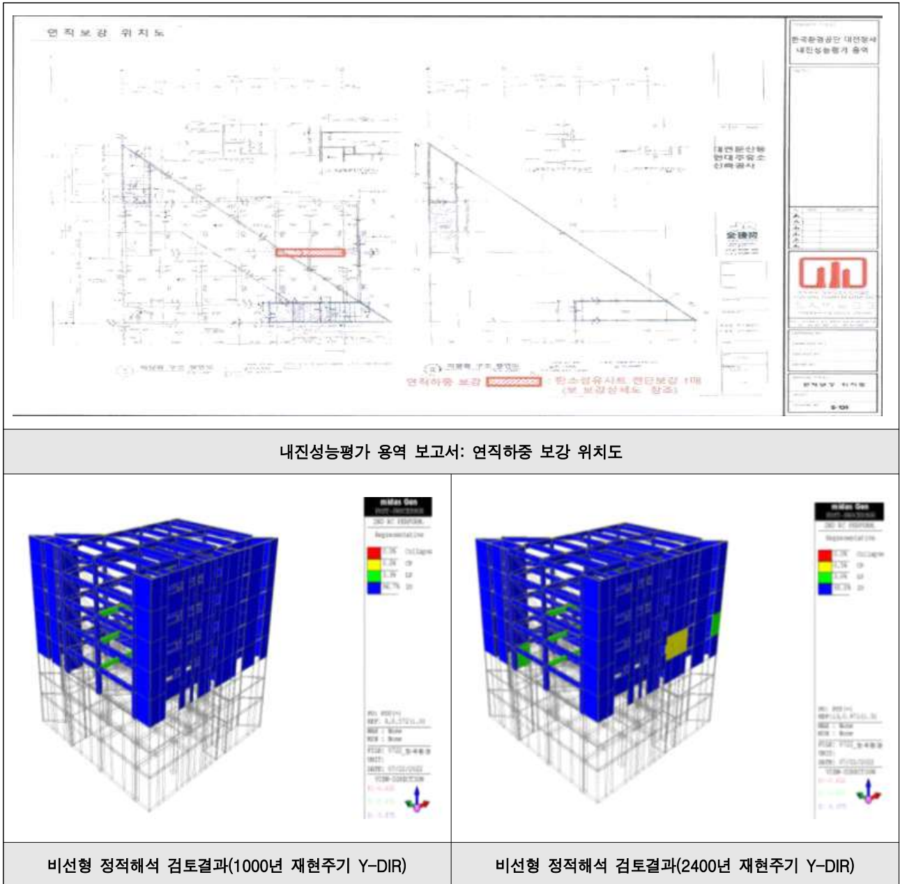
[그림 3] 연직하중 보강 위치도 및 비선형 정적해석 검토결과
